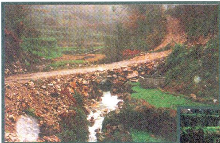
Construção de muro de suporte a estrada de Dornelas a Silva Escura.
